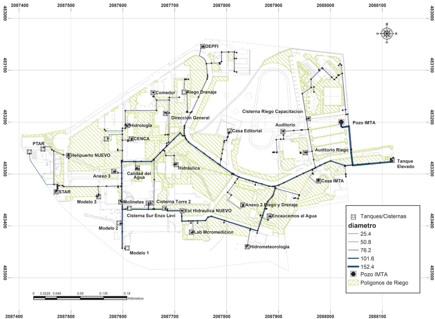
Revisión de redes de distribución en el IMTA.
