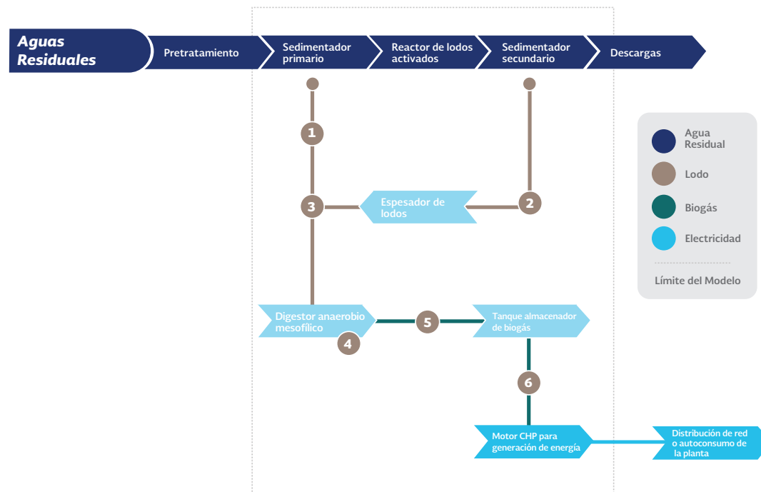
Modelo conceptual de tratamiento y cogeneración.
