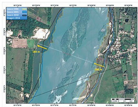
Evolución del cauce en la sección 4 del río Samaria, aguas abajo de la bifurcación.
